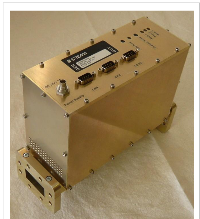
Fig. 1. HOMER Autotuner STHT 3.1.
